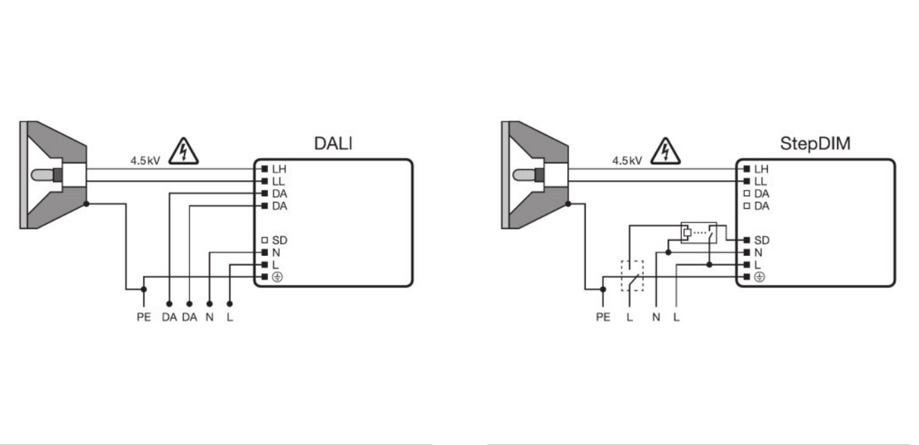
Esquema de electrificação
