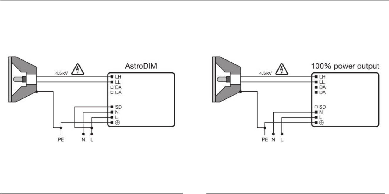
Esquema de electrificação
